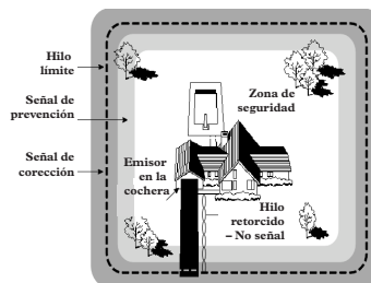
Zona de seguridad más grande Zona de advertencia más pequeña
