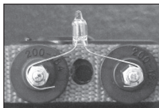
Luz de Teste nas Sondas do Receptor
