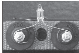
Prüflampe an den Sensoren des Empfängers
