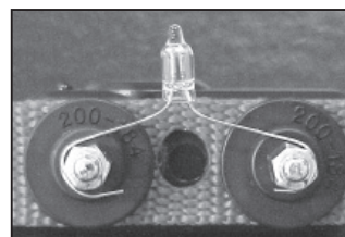
Installation de la lampe témoin sur les palpeurs
